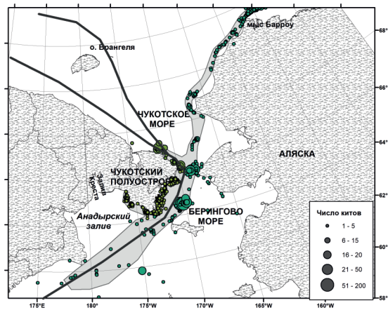
Рис. 2. Коридор весенней миграции полярных китов берингово-чукотско-бофортской популяции [16; 19; 25; 26; 28; 48]. Сплошной линией обозначен северный морской путь
